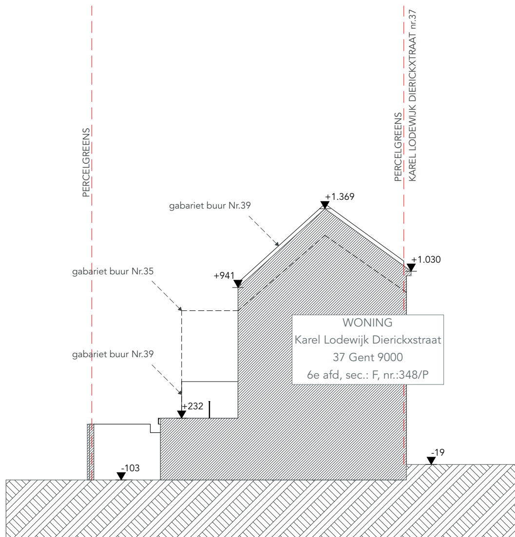
0 1 2 3 4 NT Terreinprofiel
