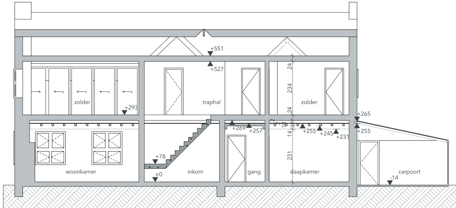
BT Doorsnede B-B
