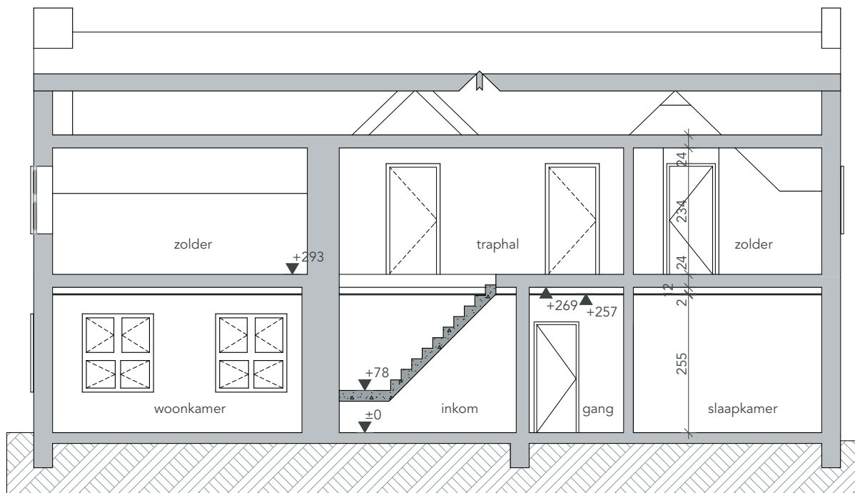
VT Doorsnede B-B
