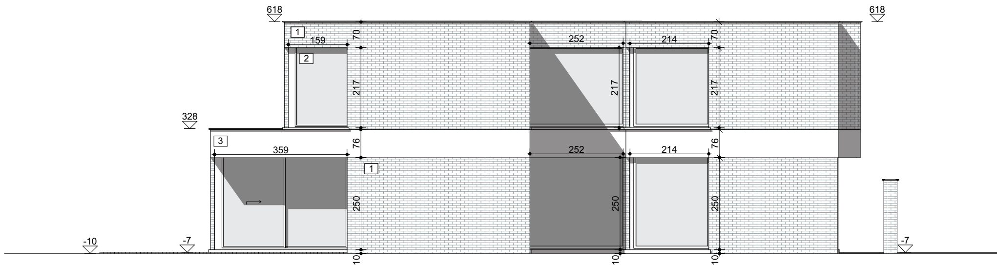
ZIJGEVEL LINKS Nieuwe toestand 1:100
