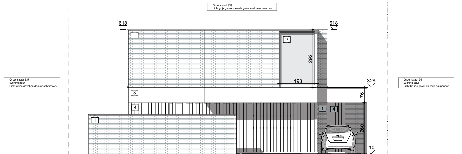
VOORGEVEL Nieuwe toestand 1:100
