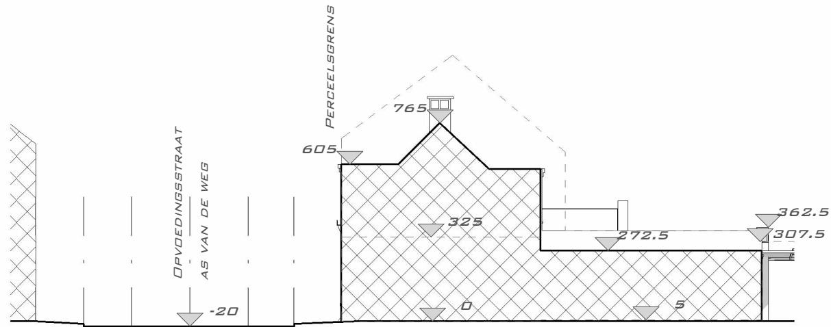
TERREINPROFIEL A BESTAAND
