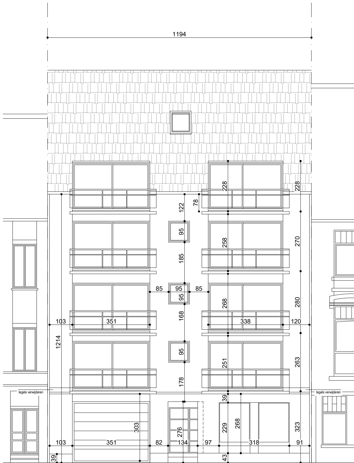
Voorgevel Bestaande toestand Schaal 1/100
