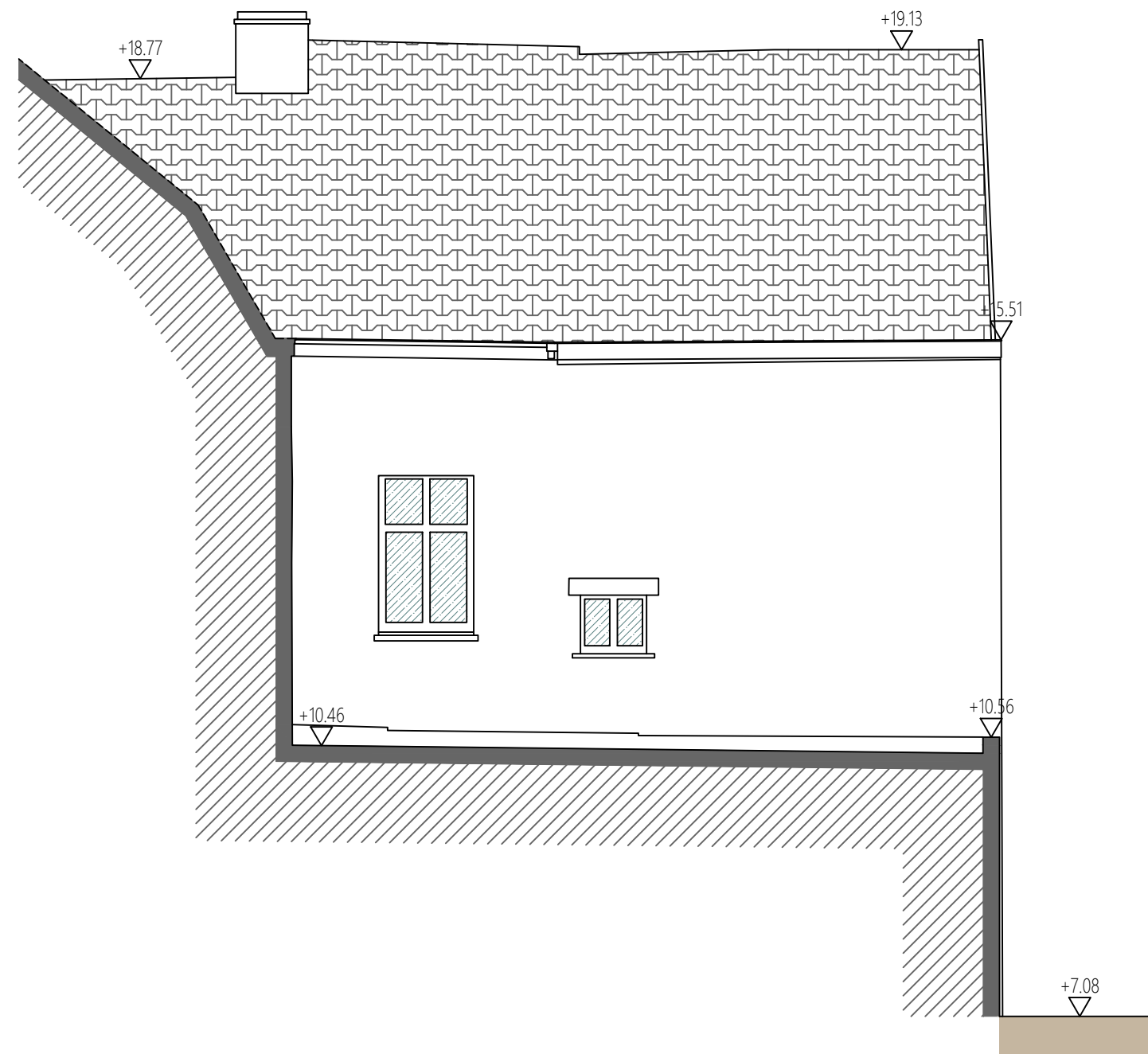
rechtergevel 2 bestaande toestand
