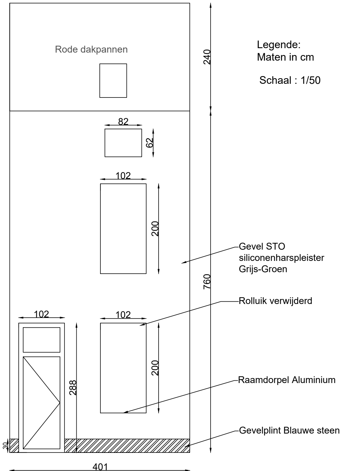
Geveltekening Nieuwe Toestand
