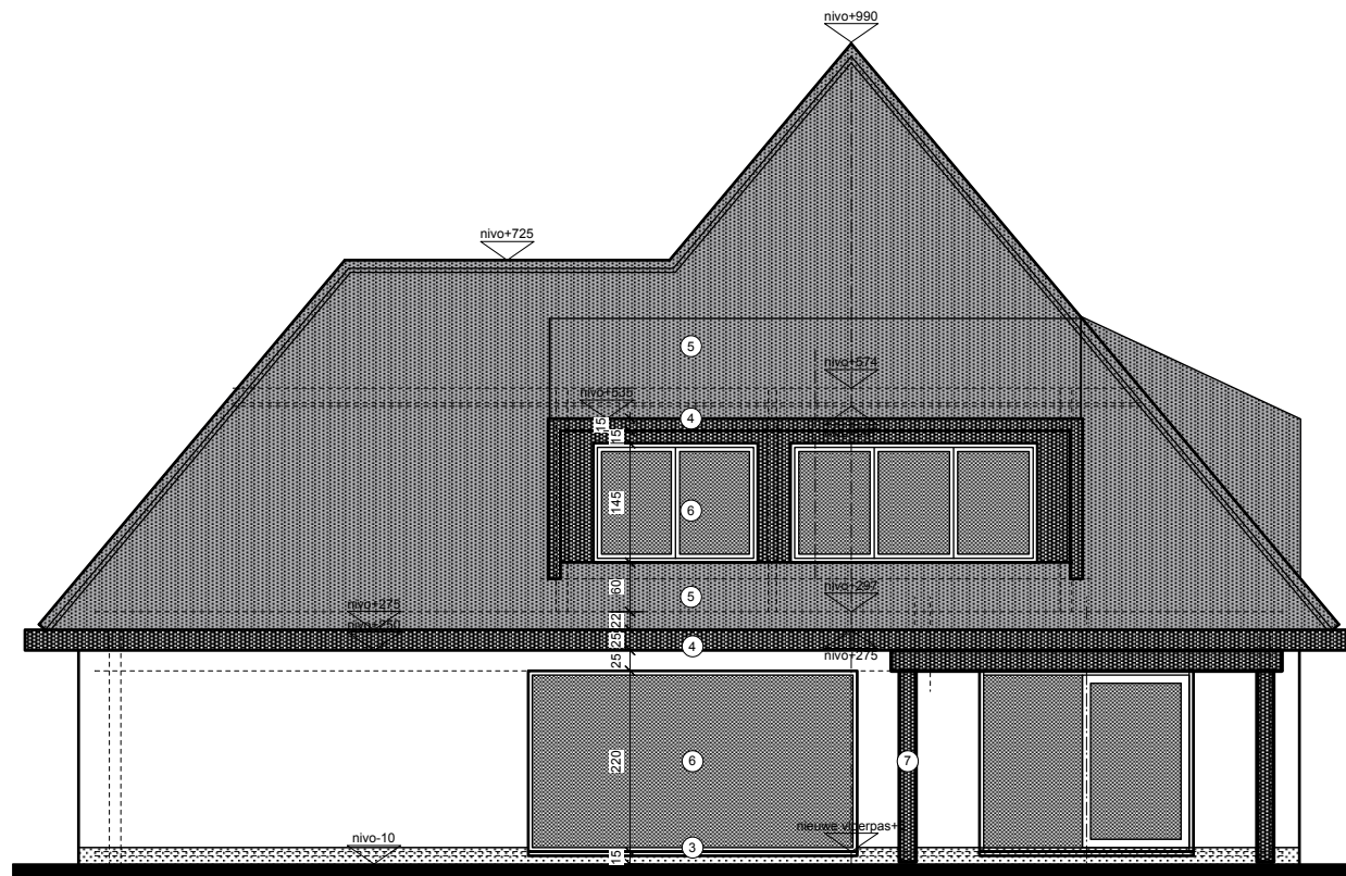
ZIJGEVEL RECHTS
