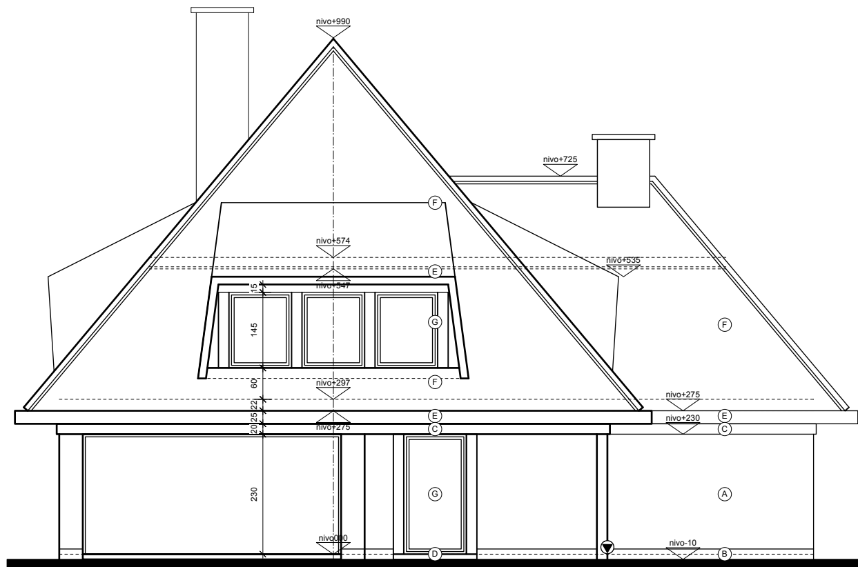
ZIJGEVEL LINKS
