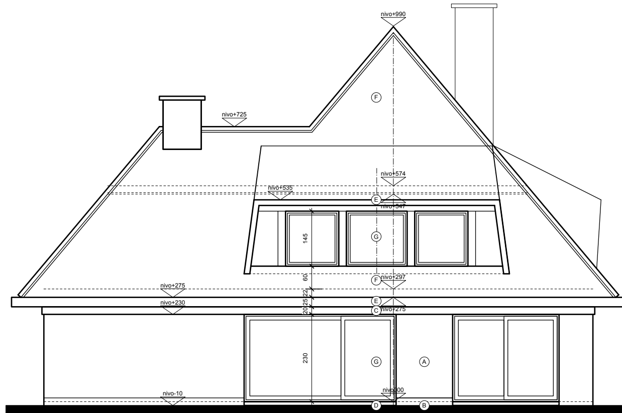
ZIJGEVEL RECHTS
