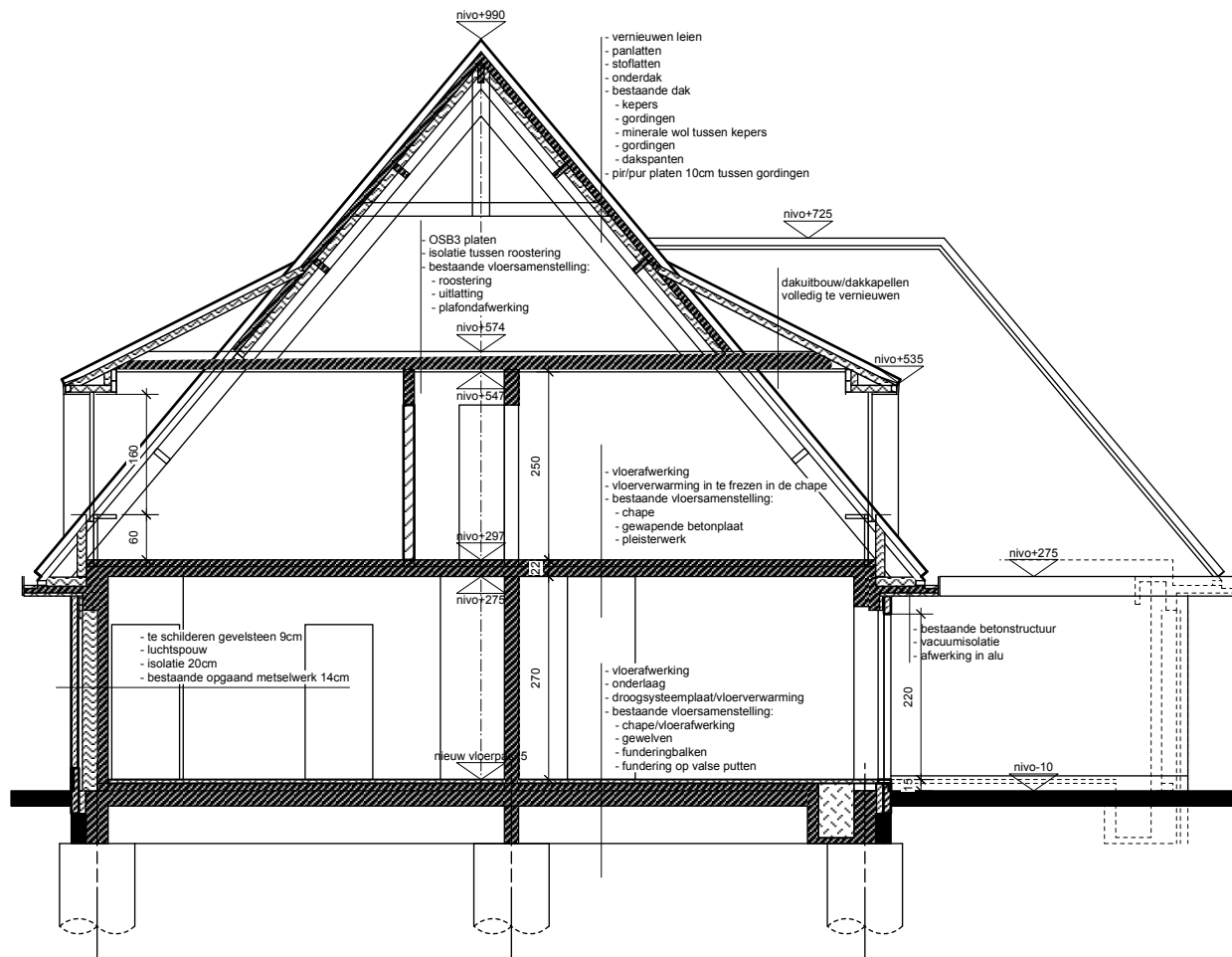
DOORSNEDE A-B
