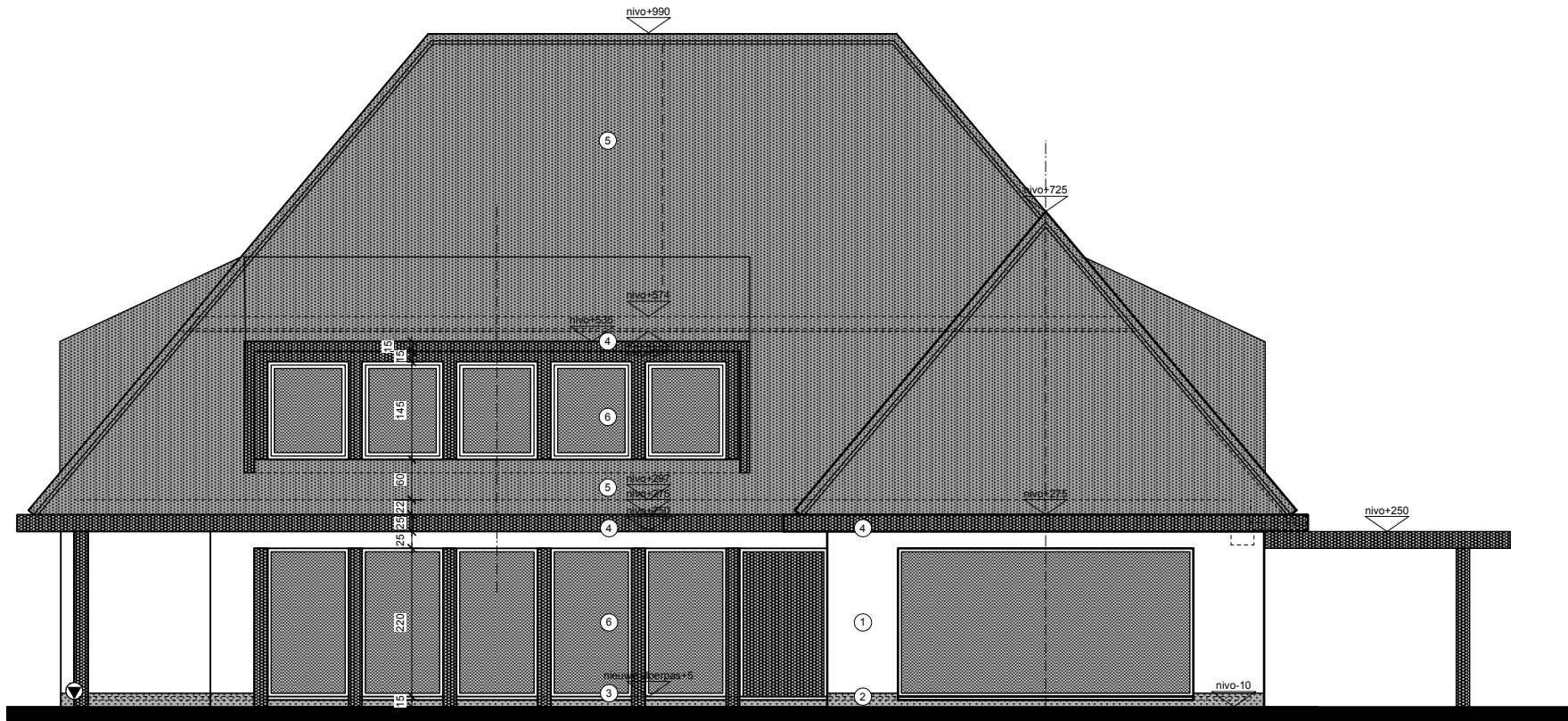
VOORGEVEL
