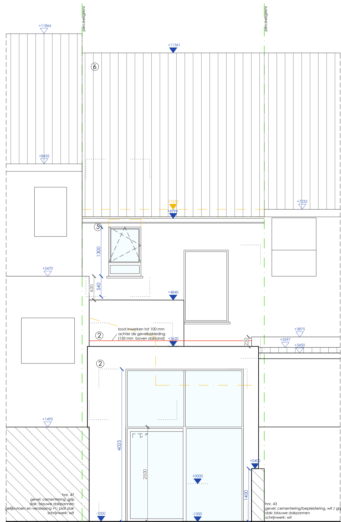
ACHTERGEVEL Nieuwe toestand BA_VERBOUWING_G_N_02_3660 Achtergevel
