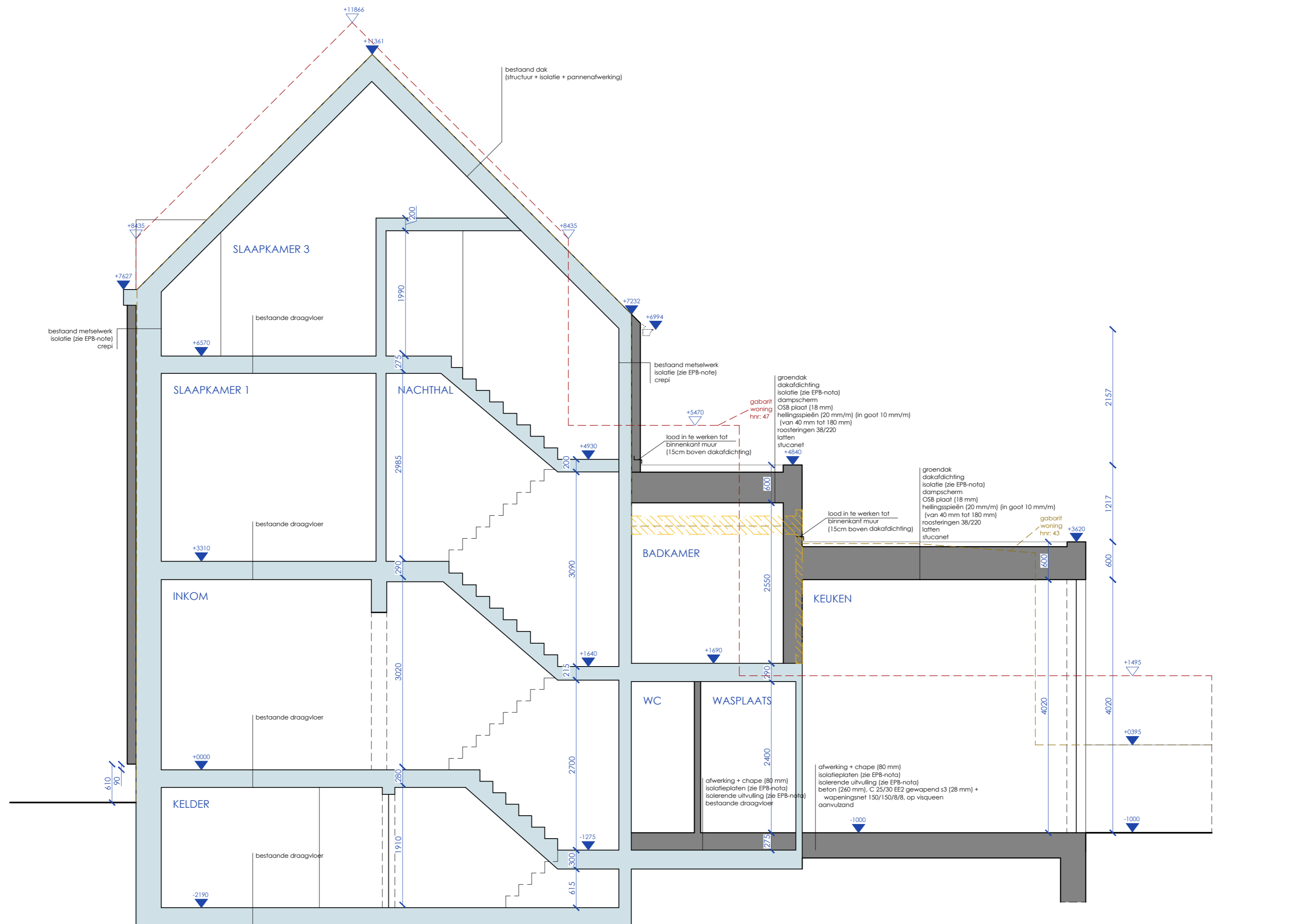
DOORSNEDE BB Nieuwe toestand BA_VERBOUWING_S_N_02_3660 Doorsnede BB
