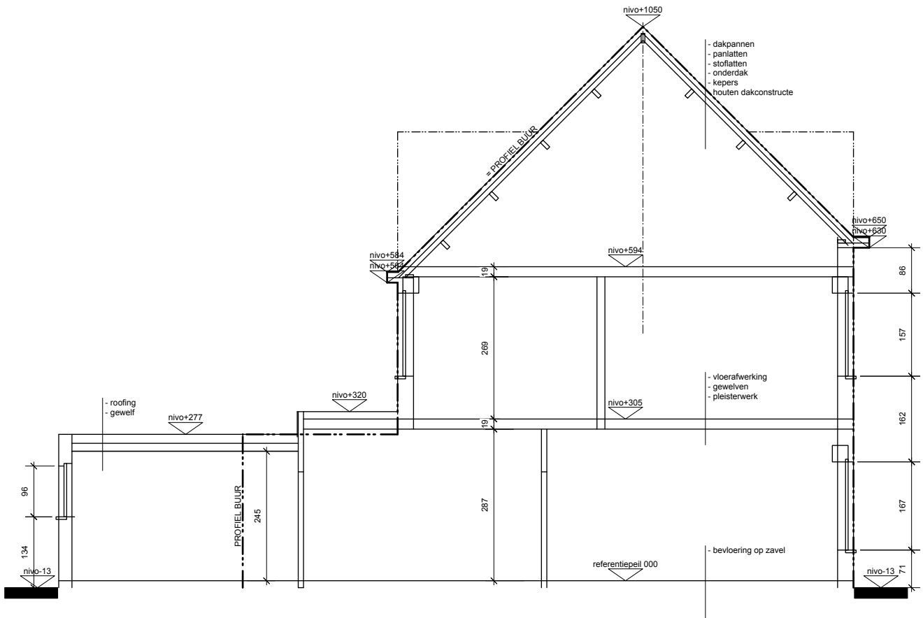
DOORSNEDE A-B
