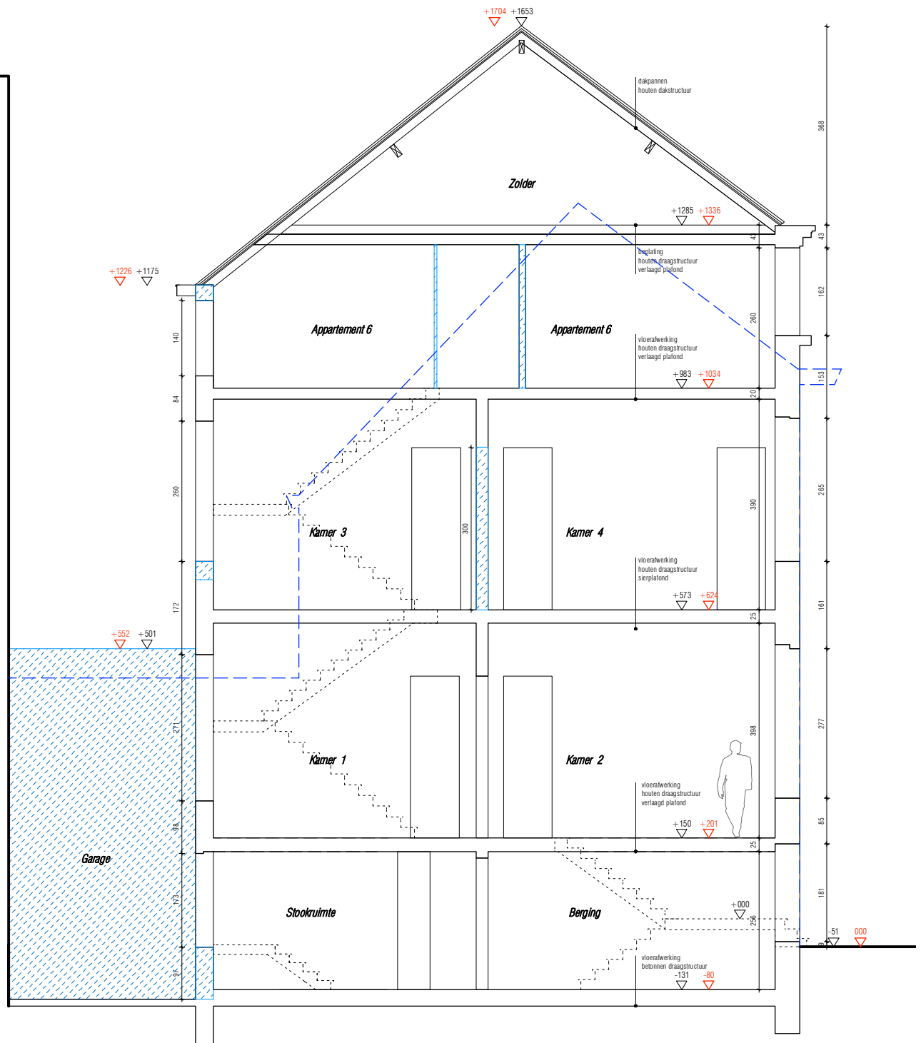
VERTICALE SNEDE
