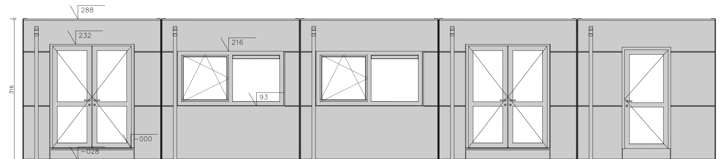
GEVEL NOORD
