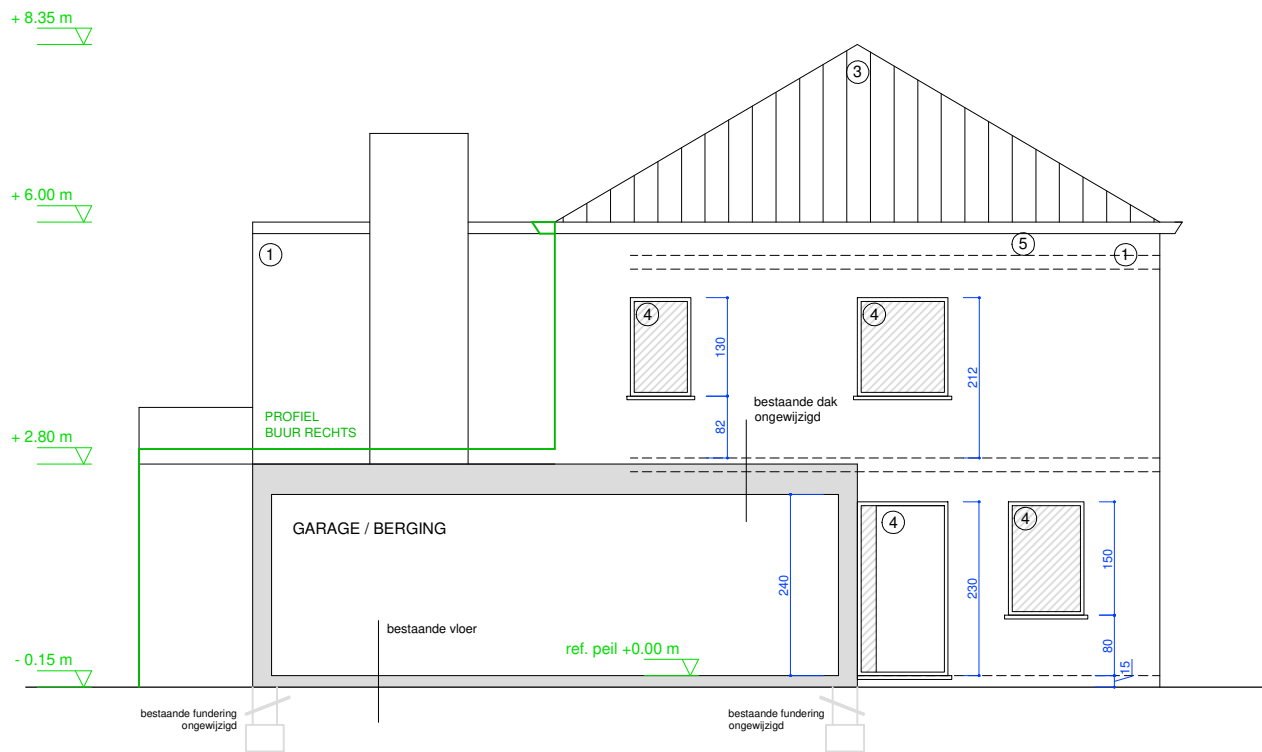
ZIJGEVEL LINKS bestaande toestand
