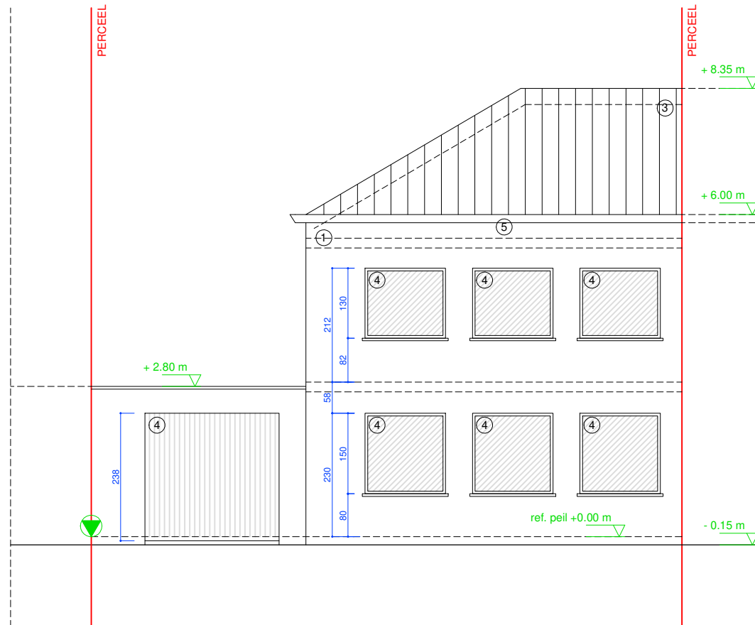
VOORGEVEL bestaande toestand
