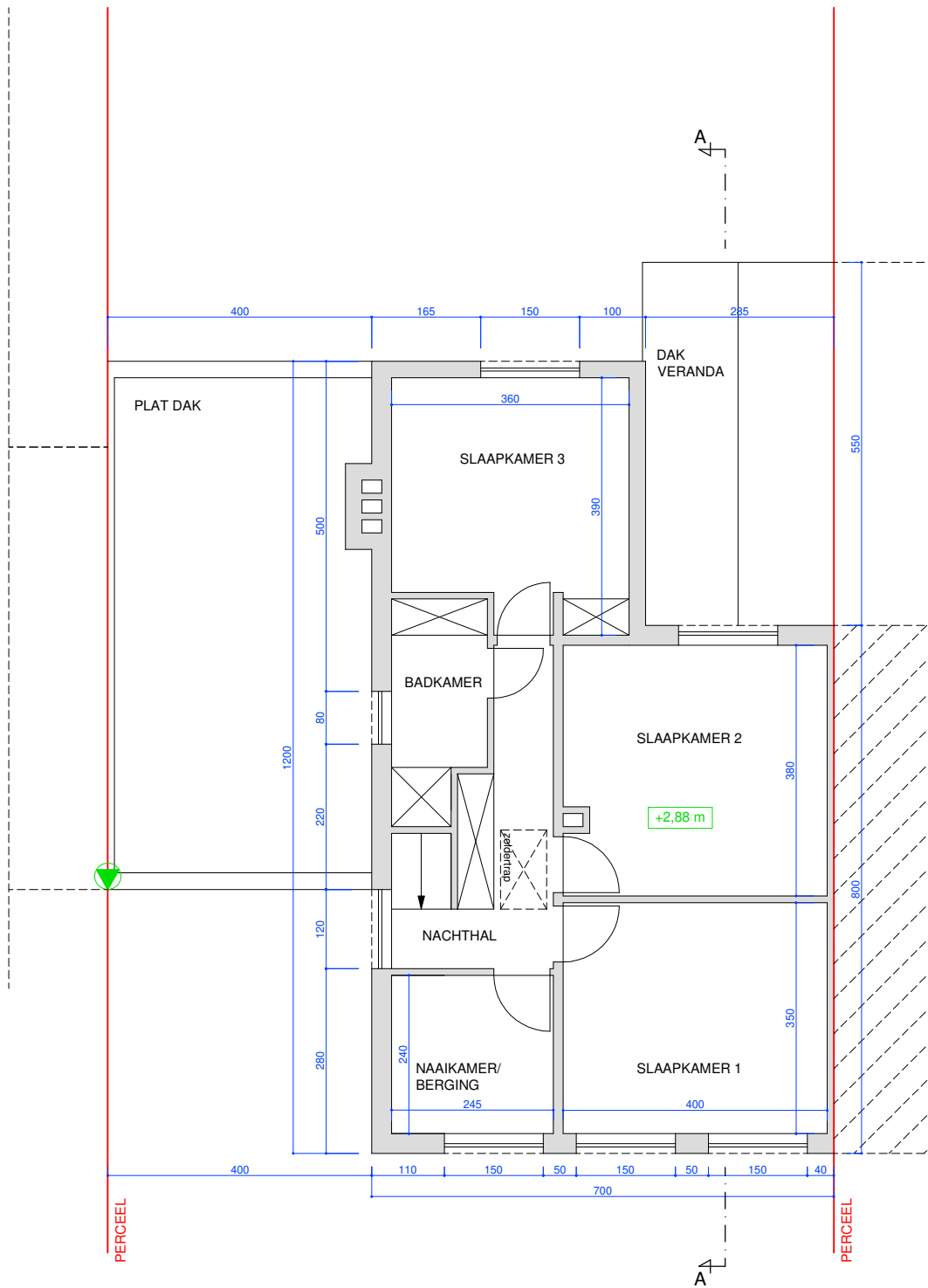
VERDIEPING bestaande toestand
