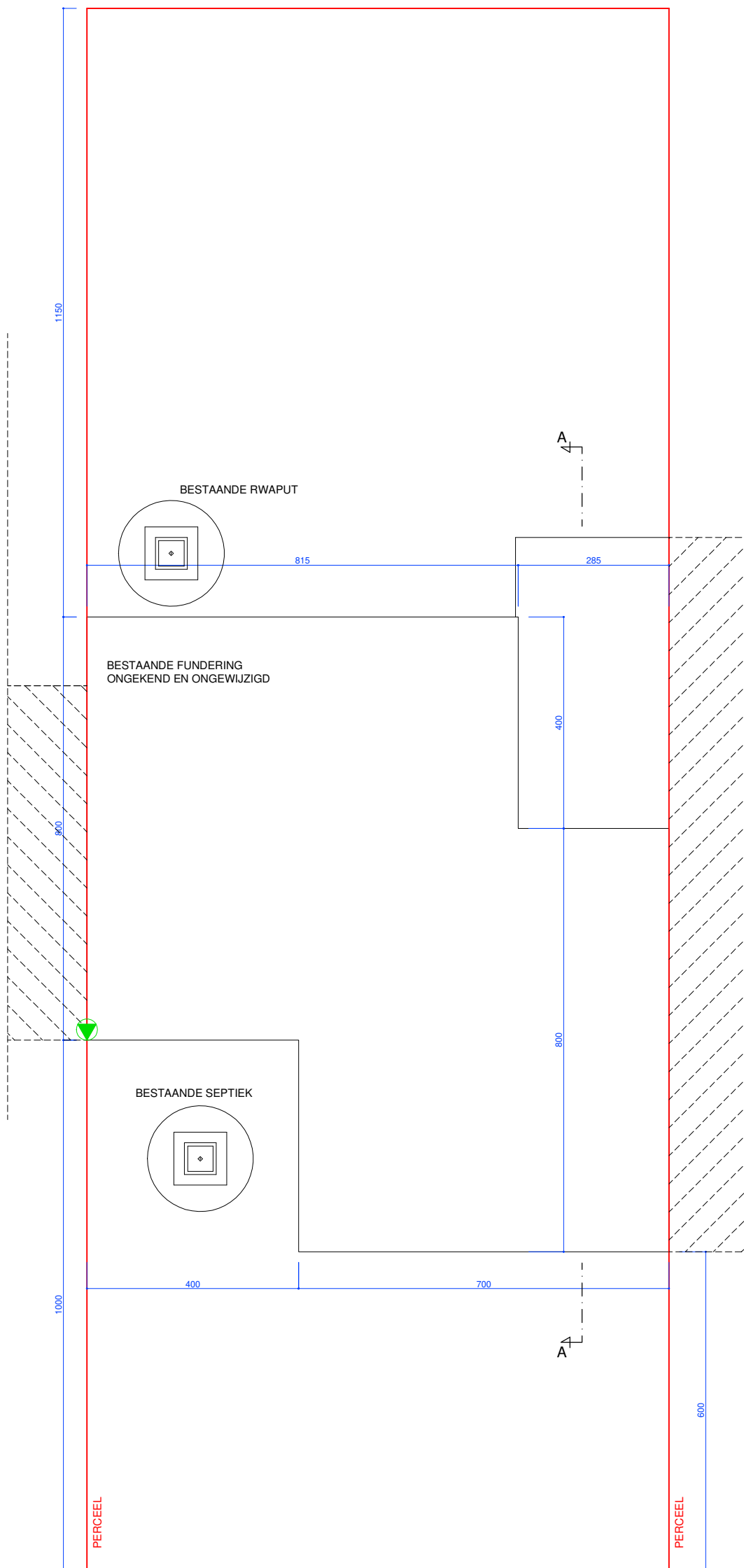
FUNDERINGS- EN RIOLERINGSPLAN bestaande toestand
