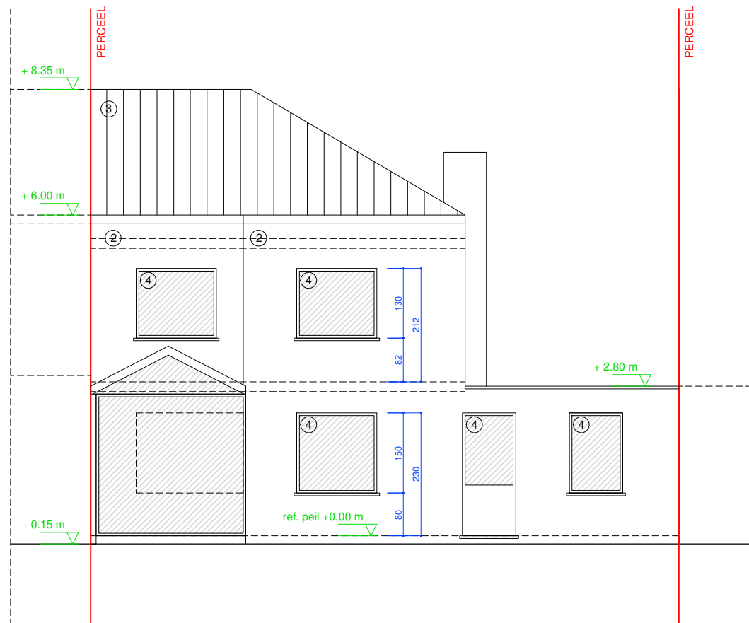
ACHTERGEVEL bestaande toestand
