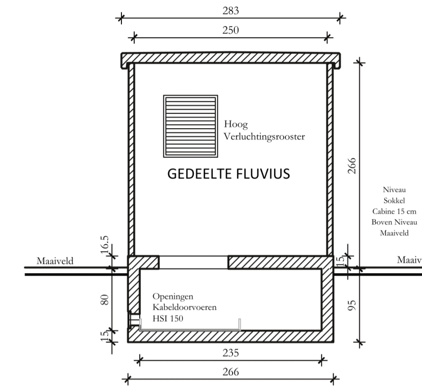
SNEDE A-A CABINE OP SCHAAL 1/50
