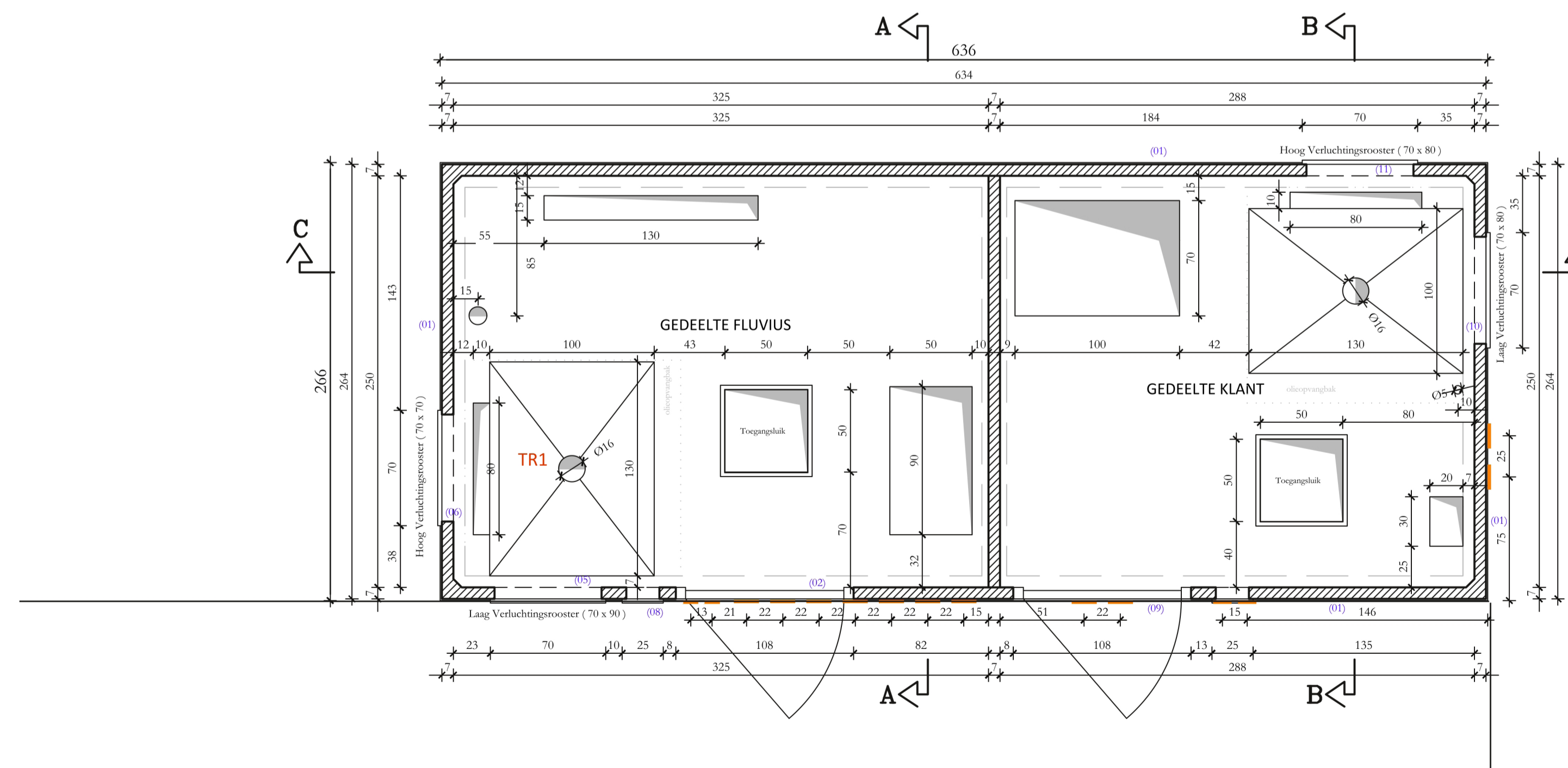
GRONDPLAN OP SCHAAL 1/25
