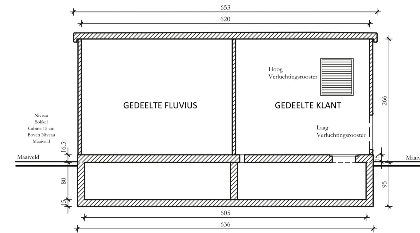
SNEDE C-C CABINE OP SCHAAL 1/50
