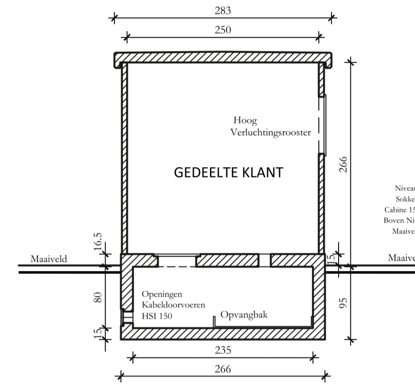
SNEDE B-B CABINE OP SCHAAL 1/50
