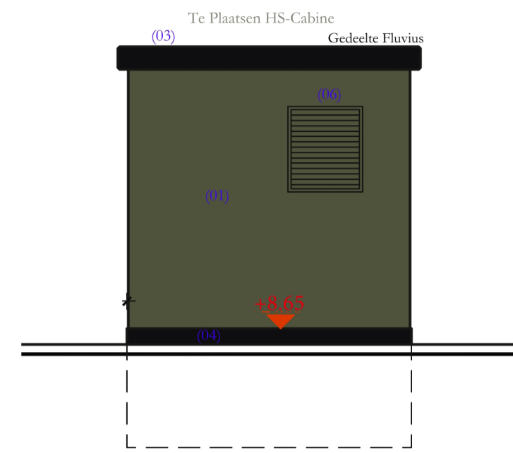
ZIJGEVEL LINKS (OOST)
