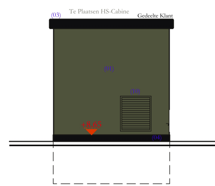
ZIJGEVEL RECHTS (WEST)
