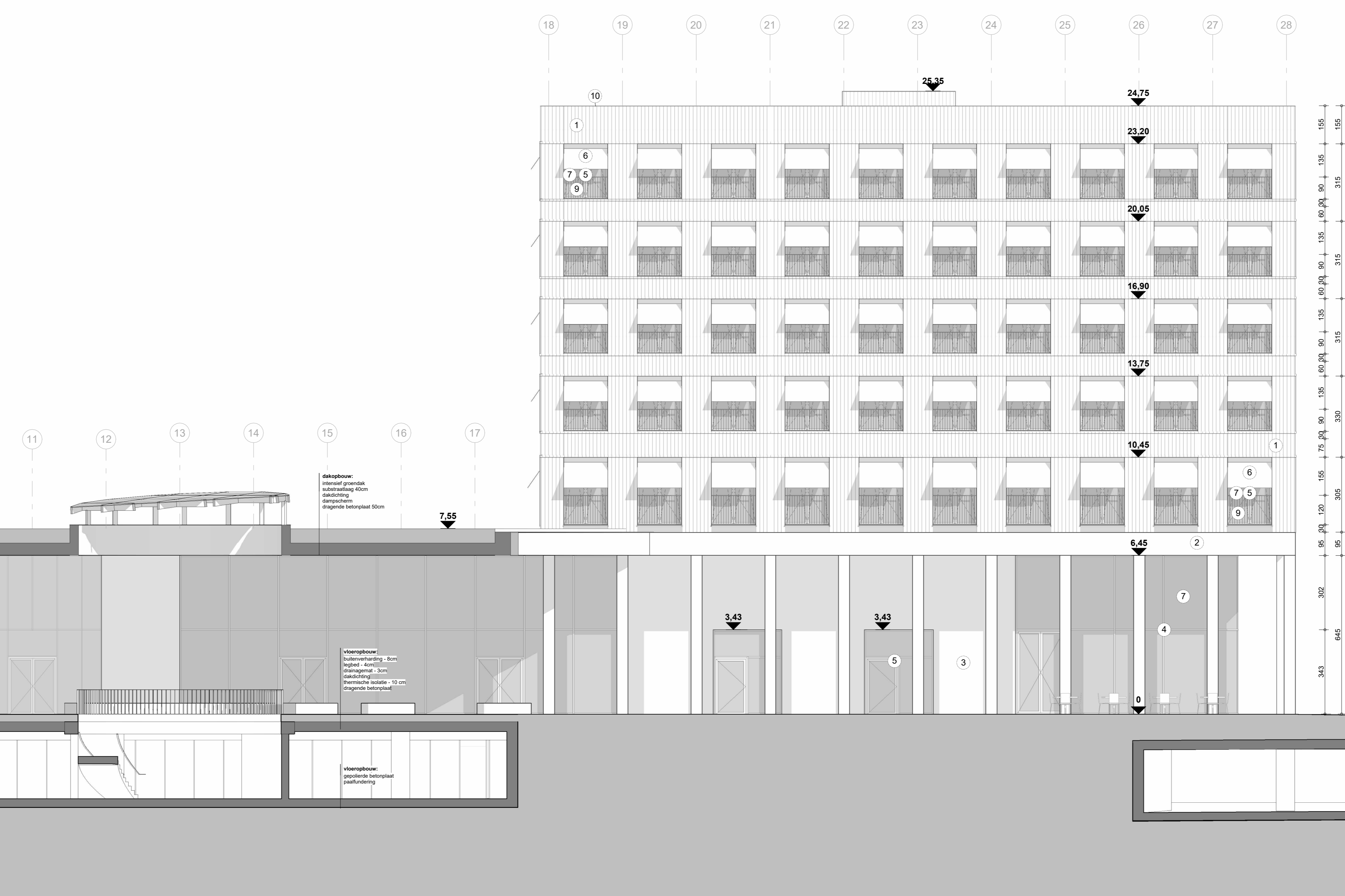
TOREN C - Zuidgevel
