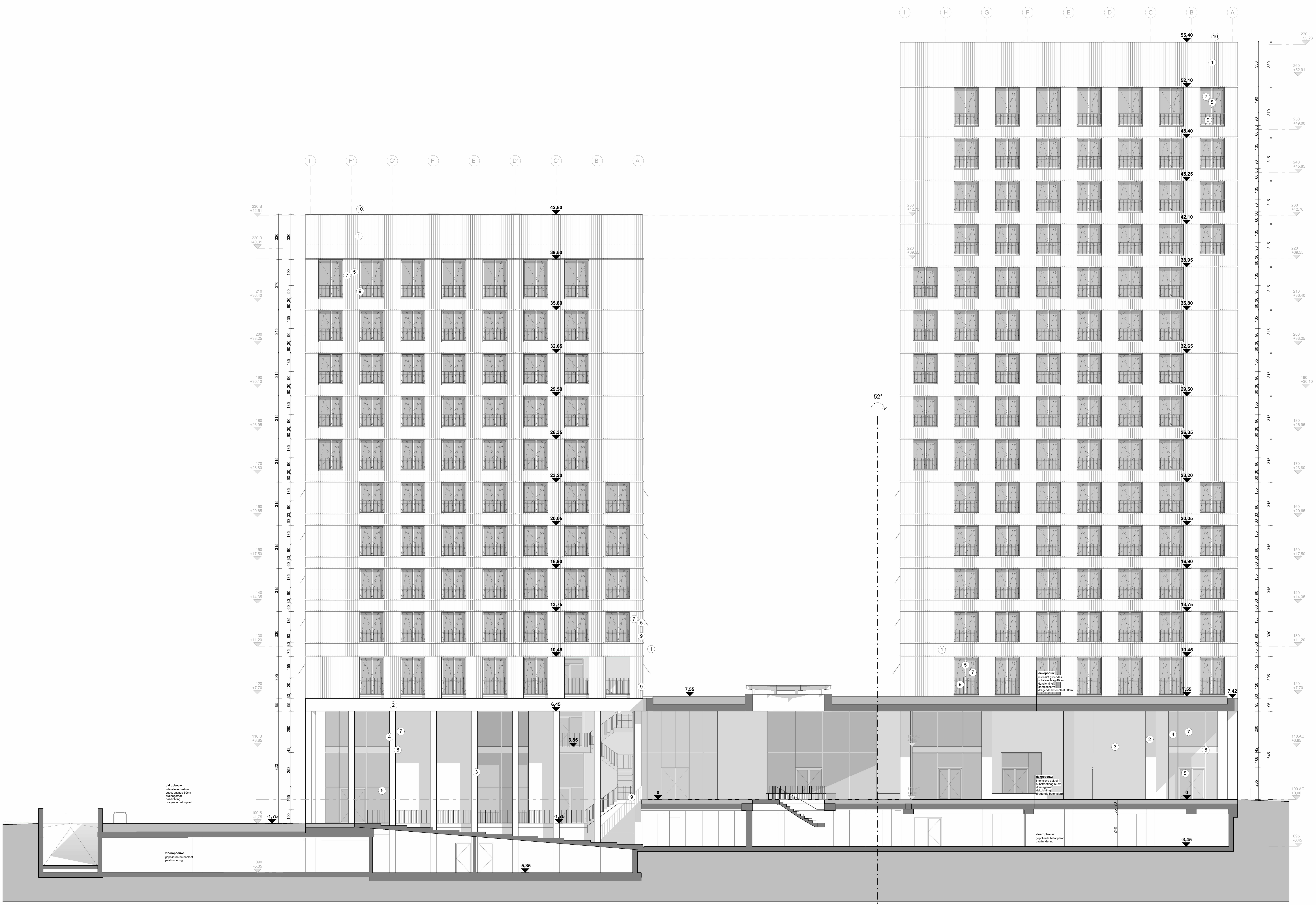
TOREN B - Noordgevel
