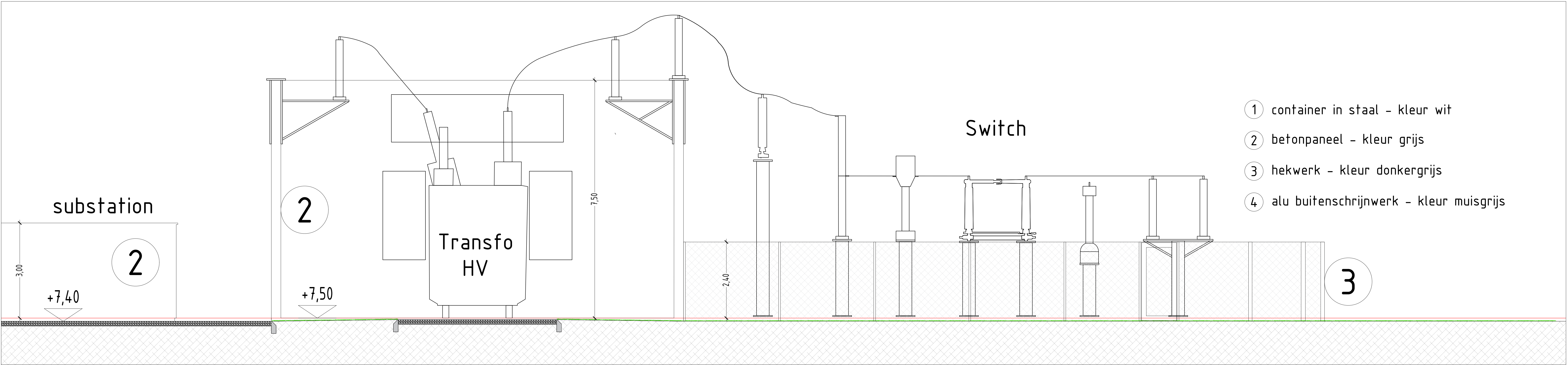
Gevel Oost - Transfo HV & Switch
