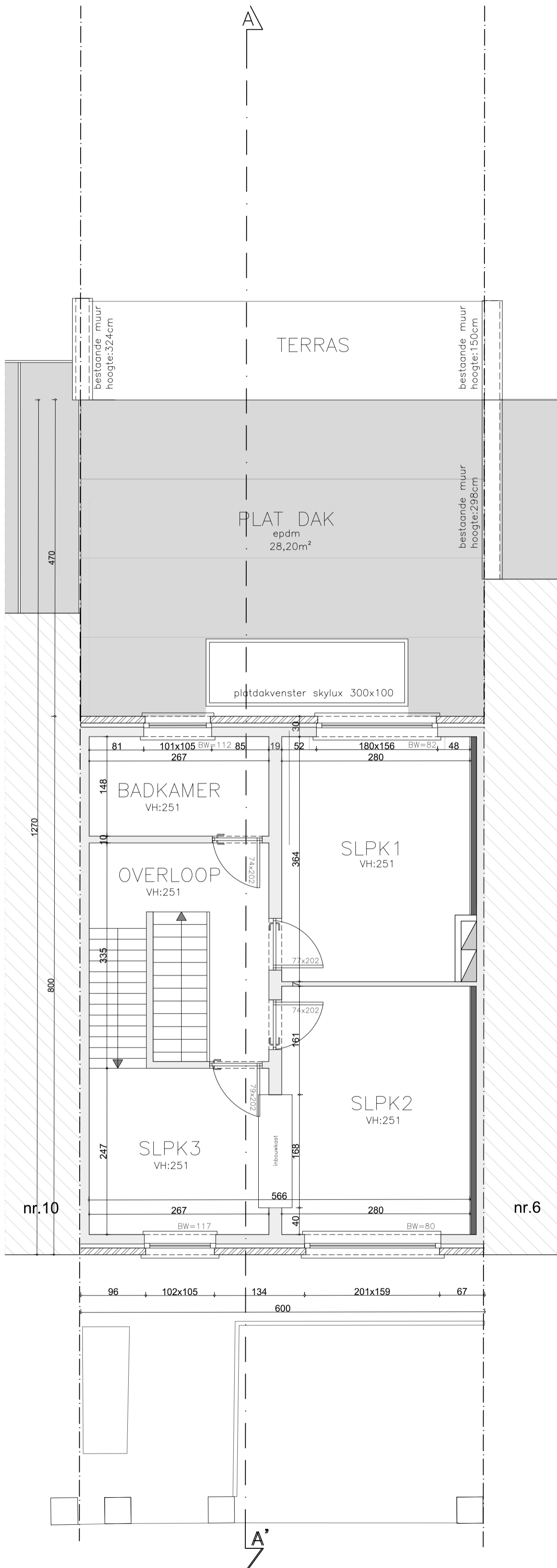
1e verdieping nieuwe toestand
