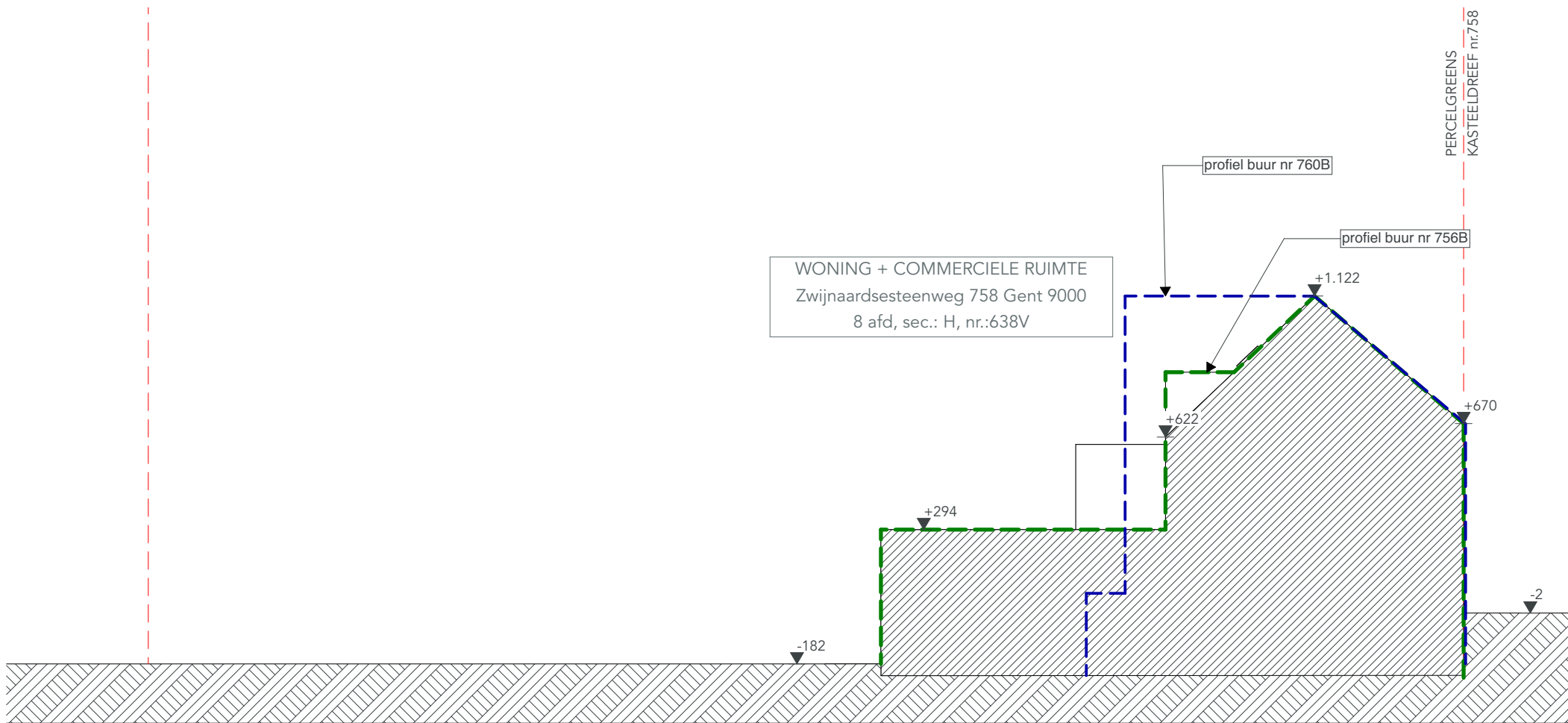
0 1 2 3 4 BT Terreinprofiel
