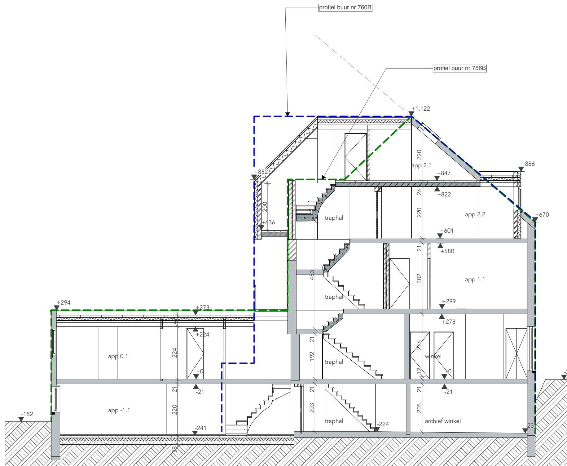
NT Doorsnede B-B
