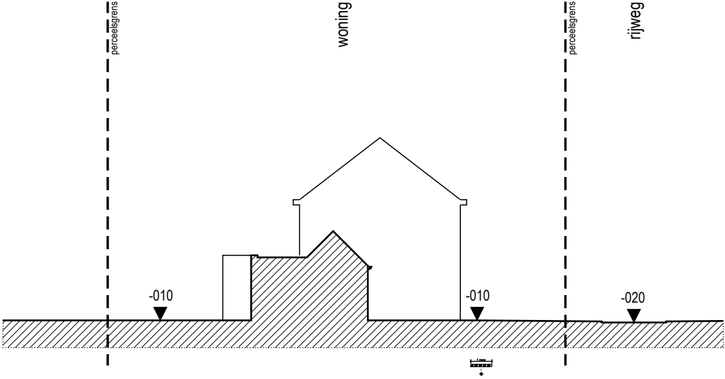
terreinprofiel AA
