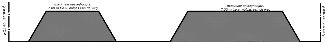
Terreinprofiel T3 nieuw - schaal 1/500
