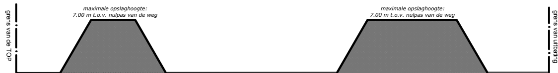
Terreinprofiel T4 nieuw - schaal 1/500
