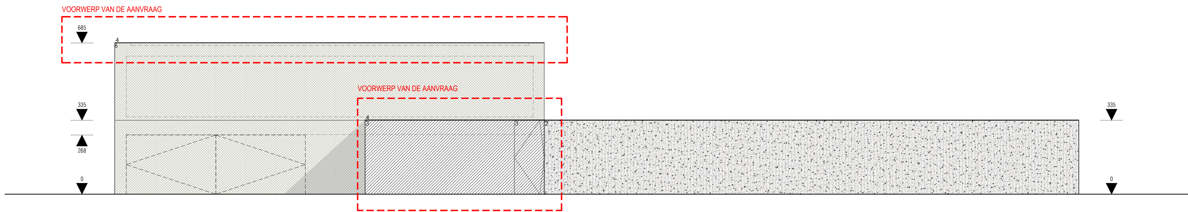
Noordwest gevel
