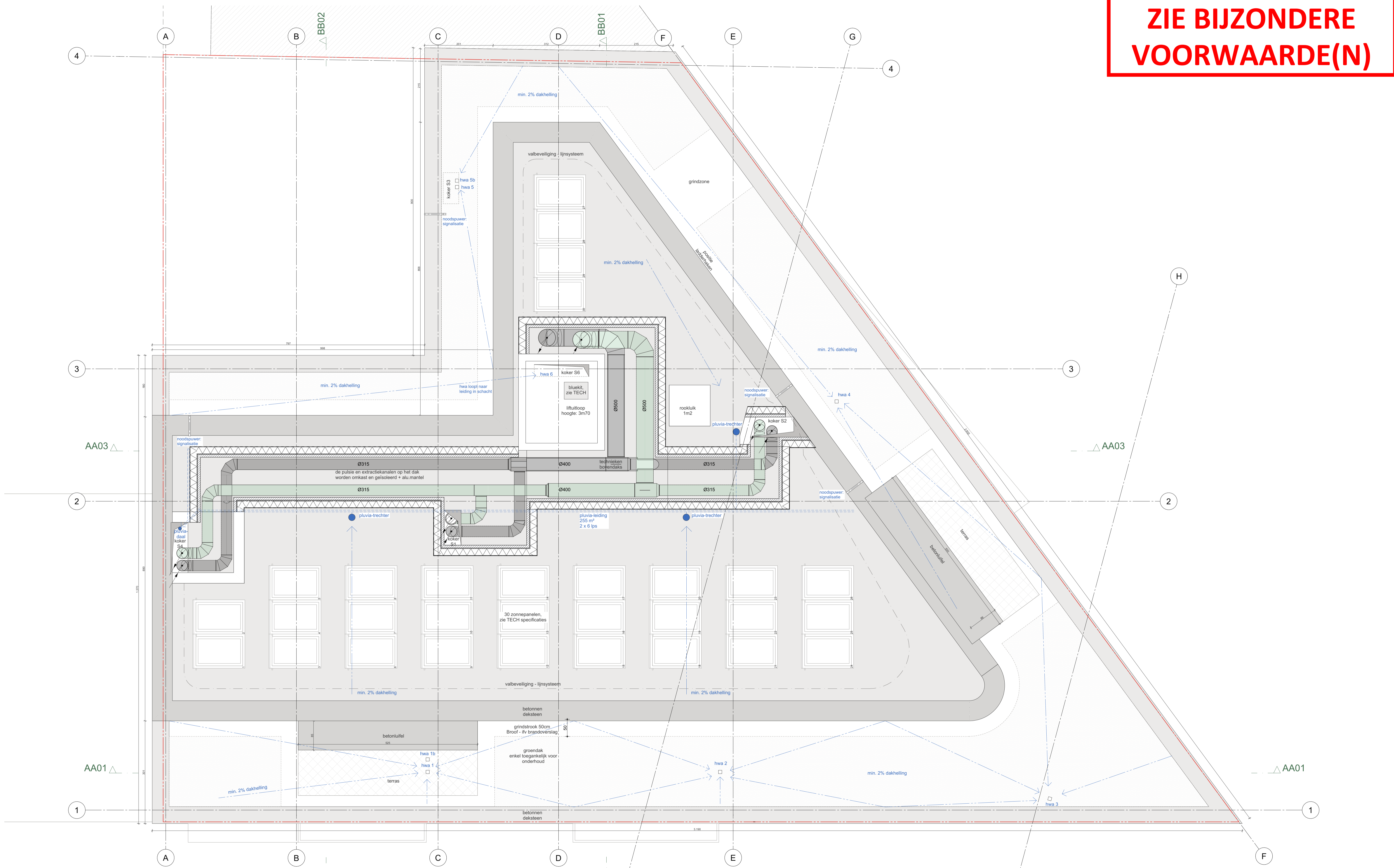
Plan dak +05 1:50 maatvoering cm
