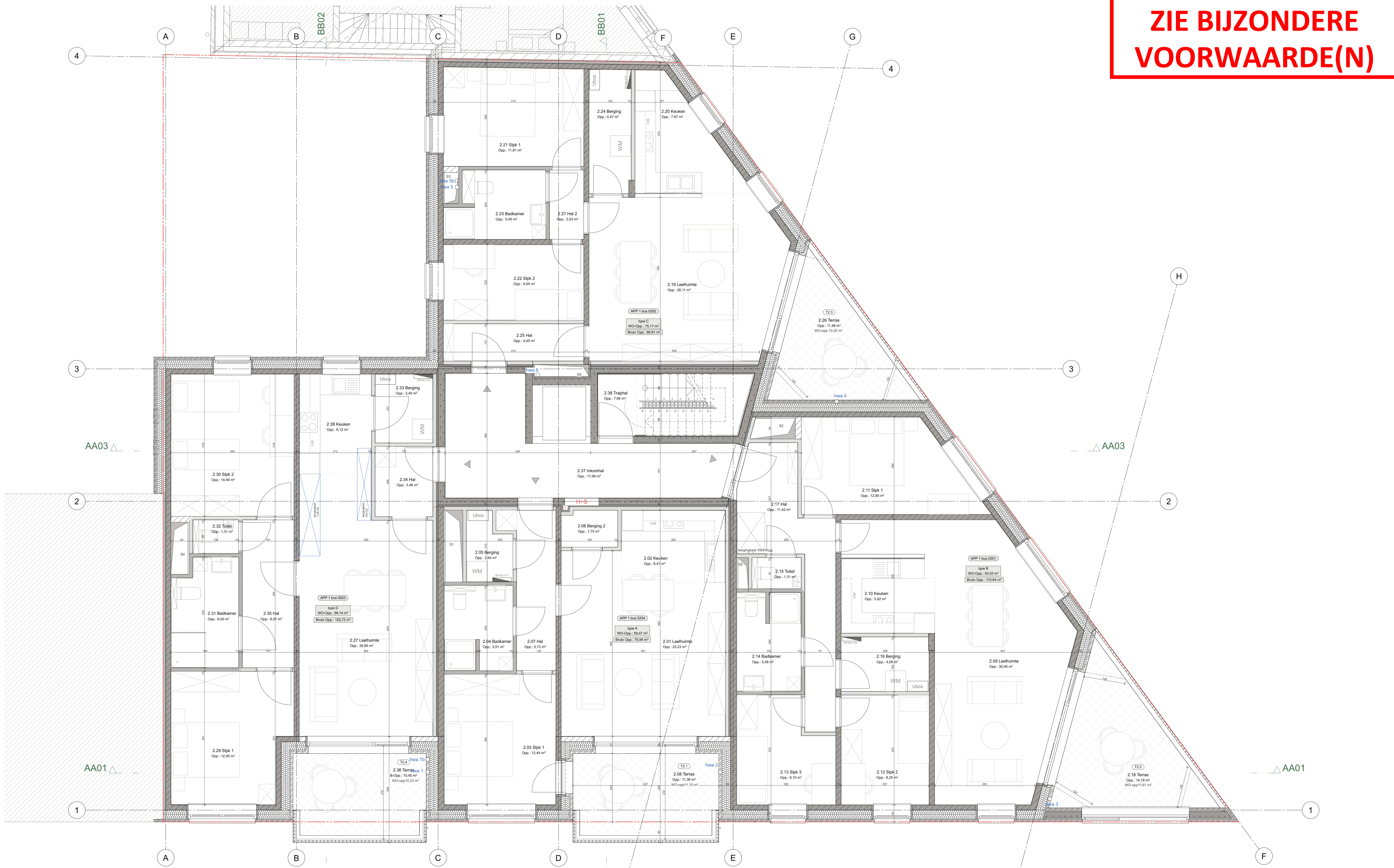
Plan+02 1:50 maatvoering cm
