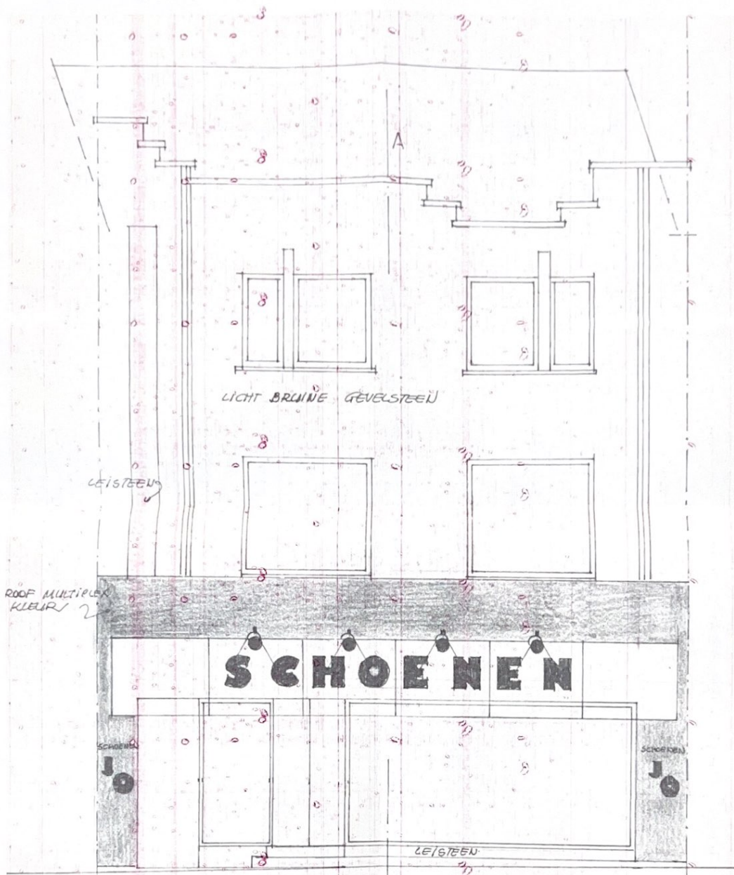
VOORGEVEL-ONTWERP VERGUNDE TOESTAND
