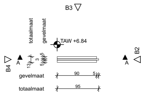
Bovenaanzicht
