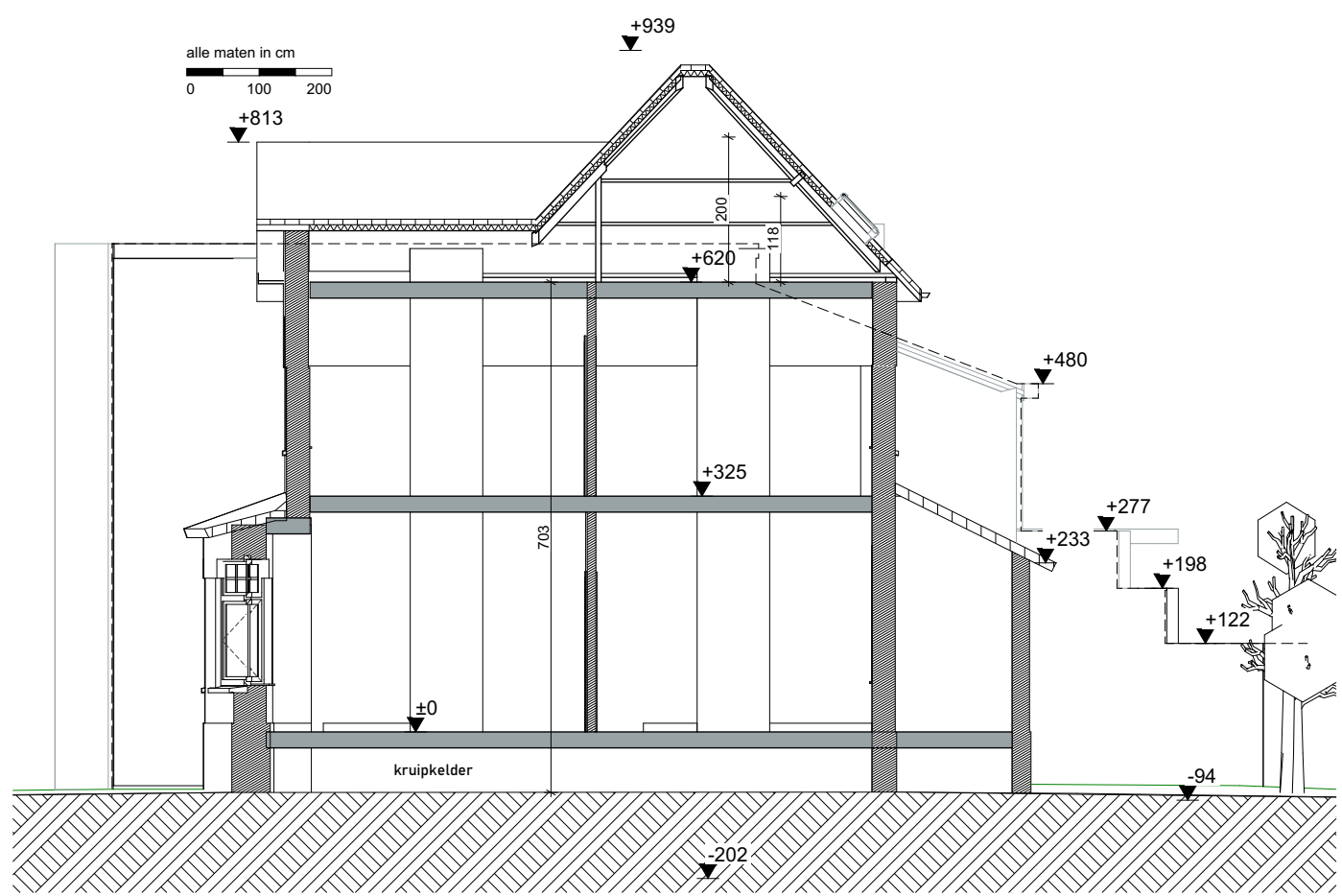
Doorsnede A-A
