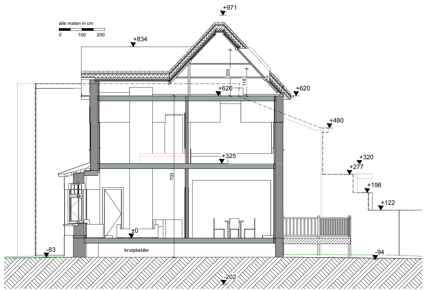
Doorsnede A-A
