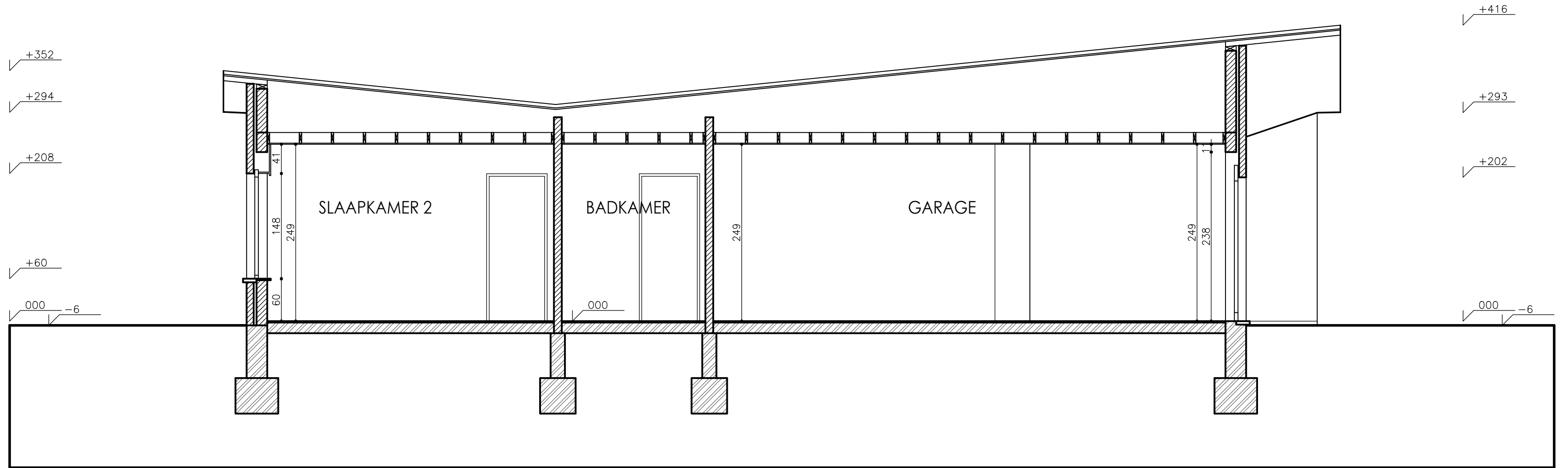
DOORSNEDE AB
