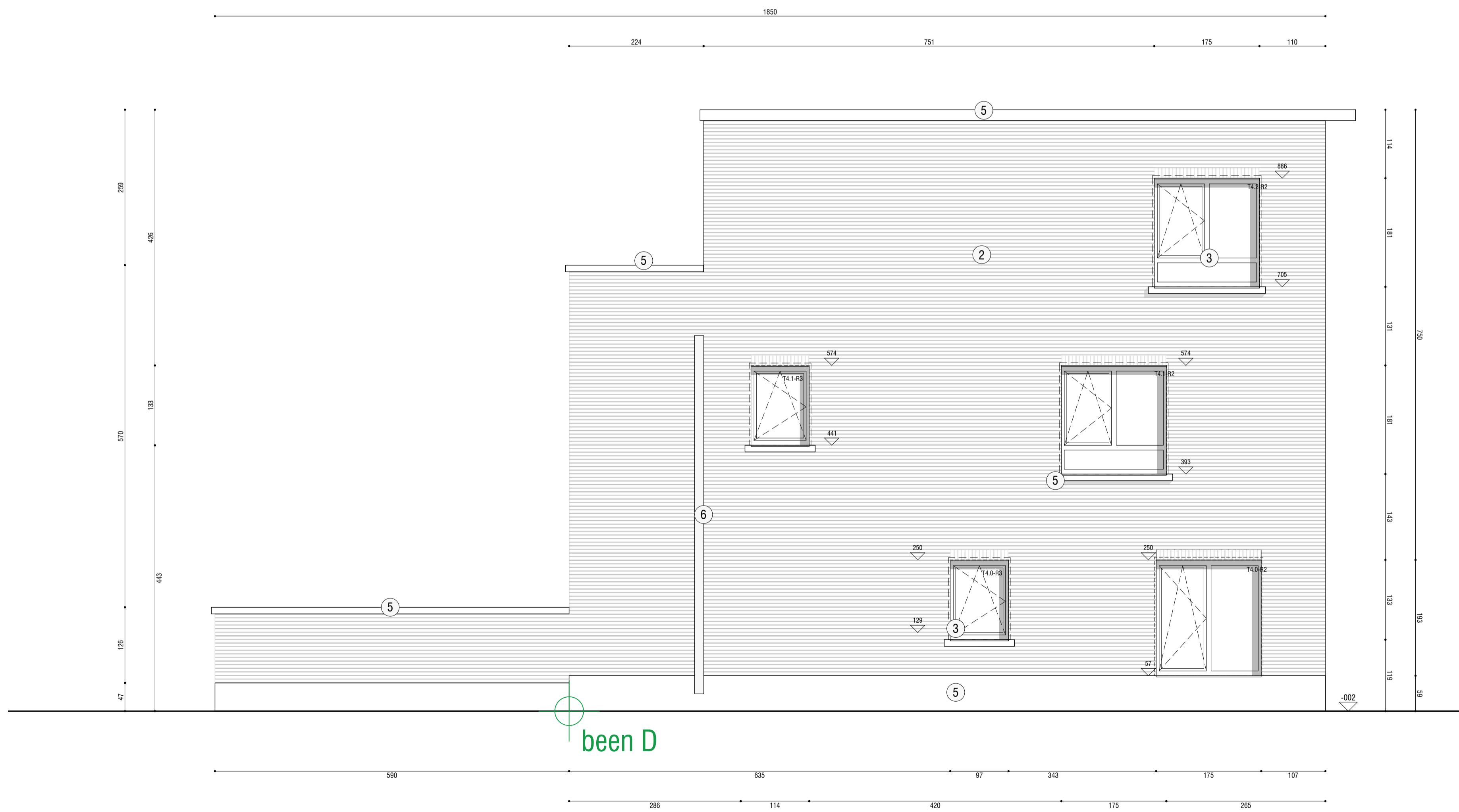
aanzicht achtergevel_D
