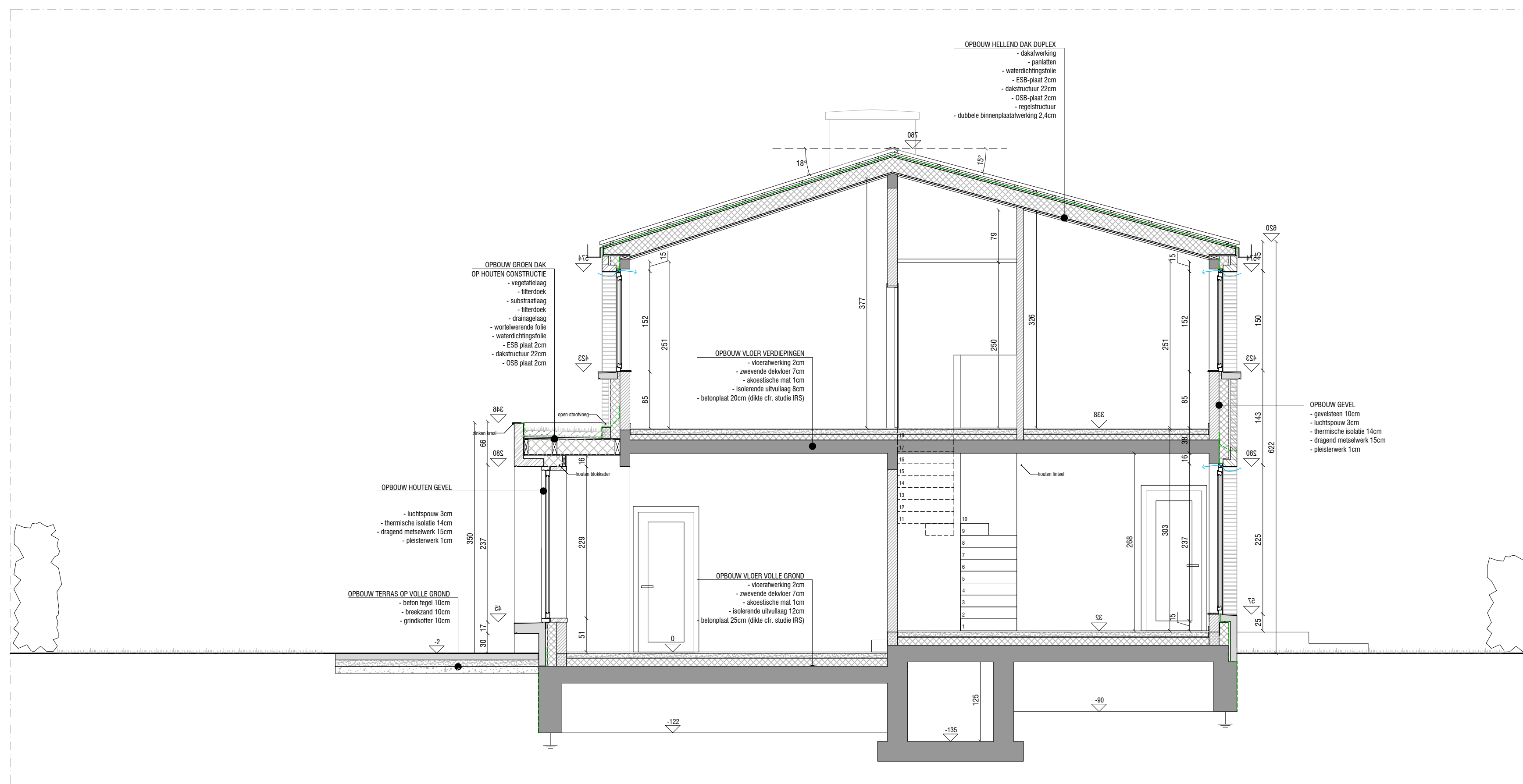
snede BB_C
