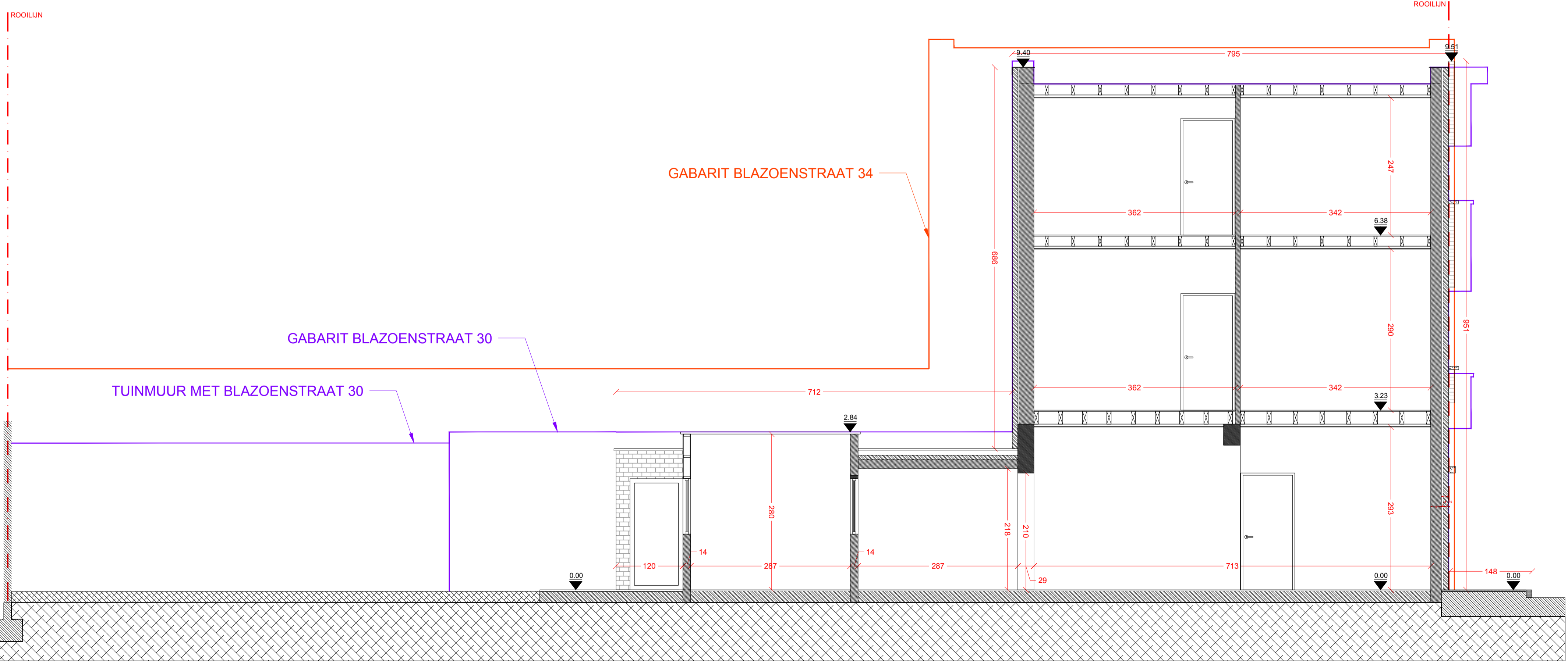
BLAZOENSTRAAT 32 LANGSE SNEDE VERGUNDE TOESTAND
