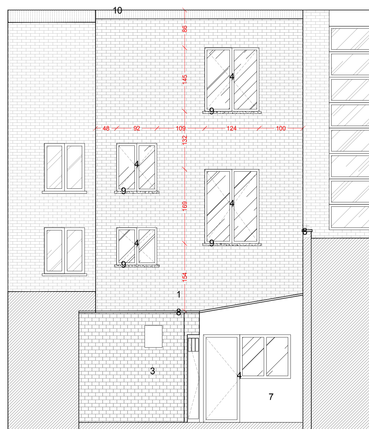
BLAZOENSTRAAT 32 ACHTERGEVEL VERGUNDE TOESTAND
