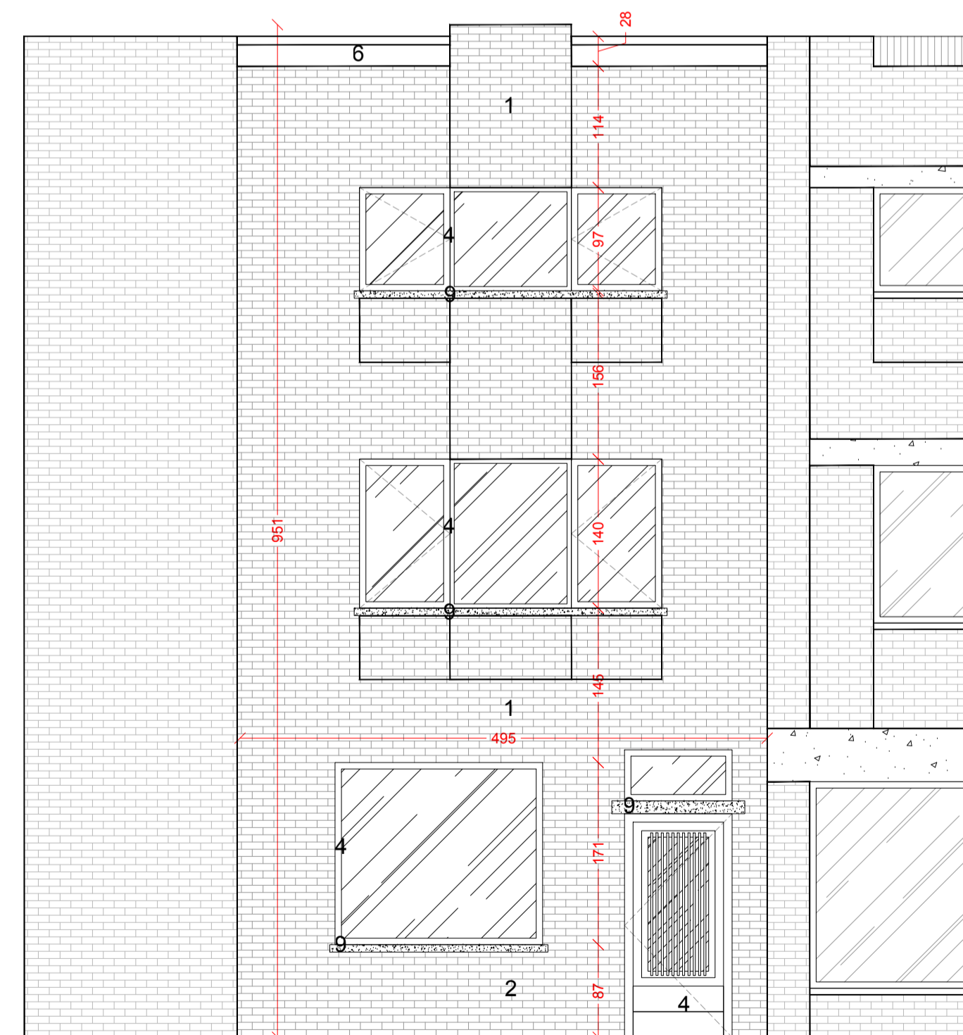
BLAZOENSTRAAT 32 VOORGEVEL VERGUNDE TOESTAND
