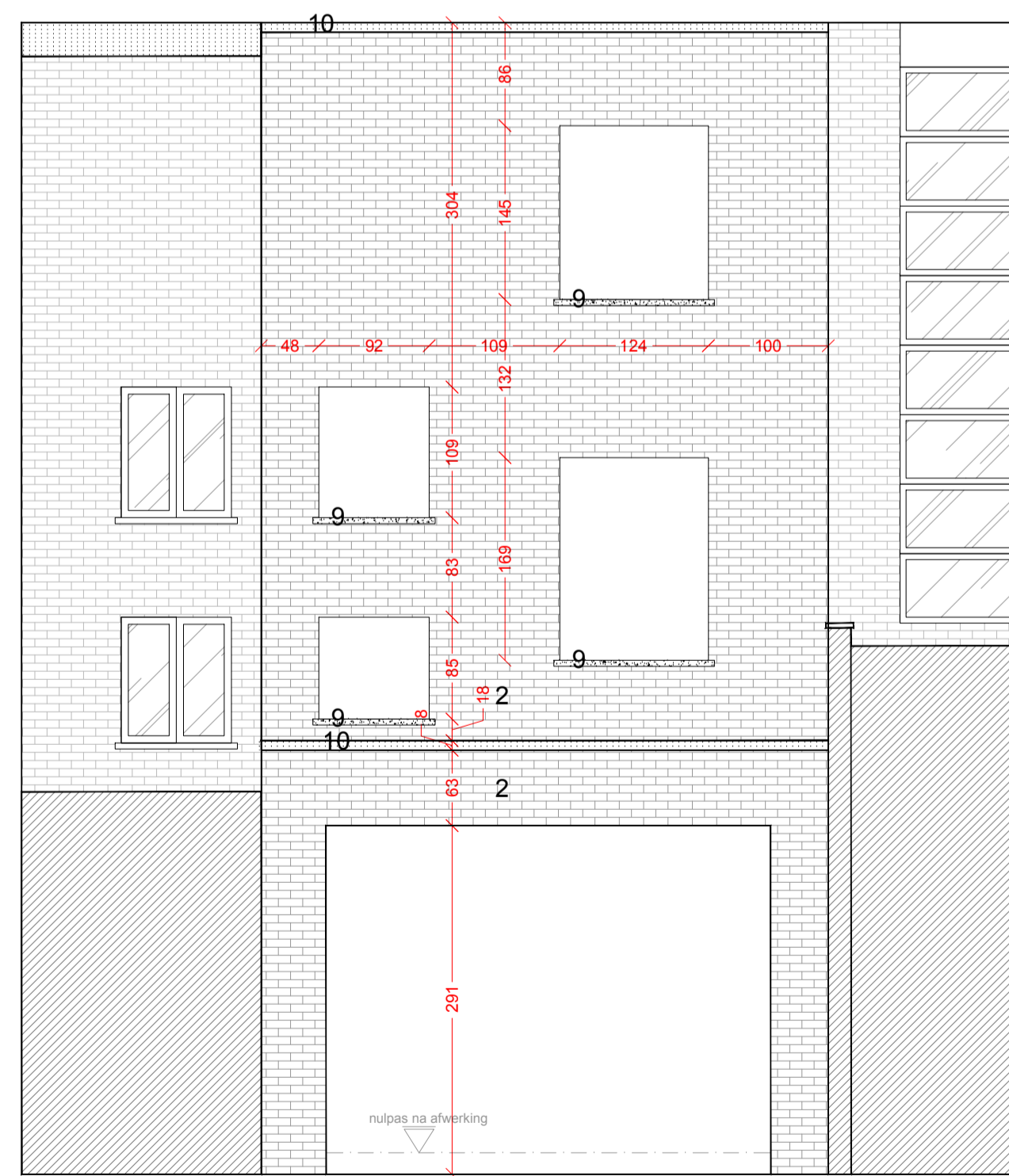
BLAZOENSTRAAT 32 ACHTERGEVEL BESTAANDE TOESTAND
