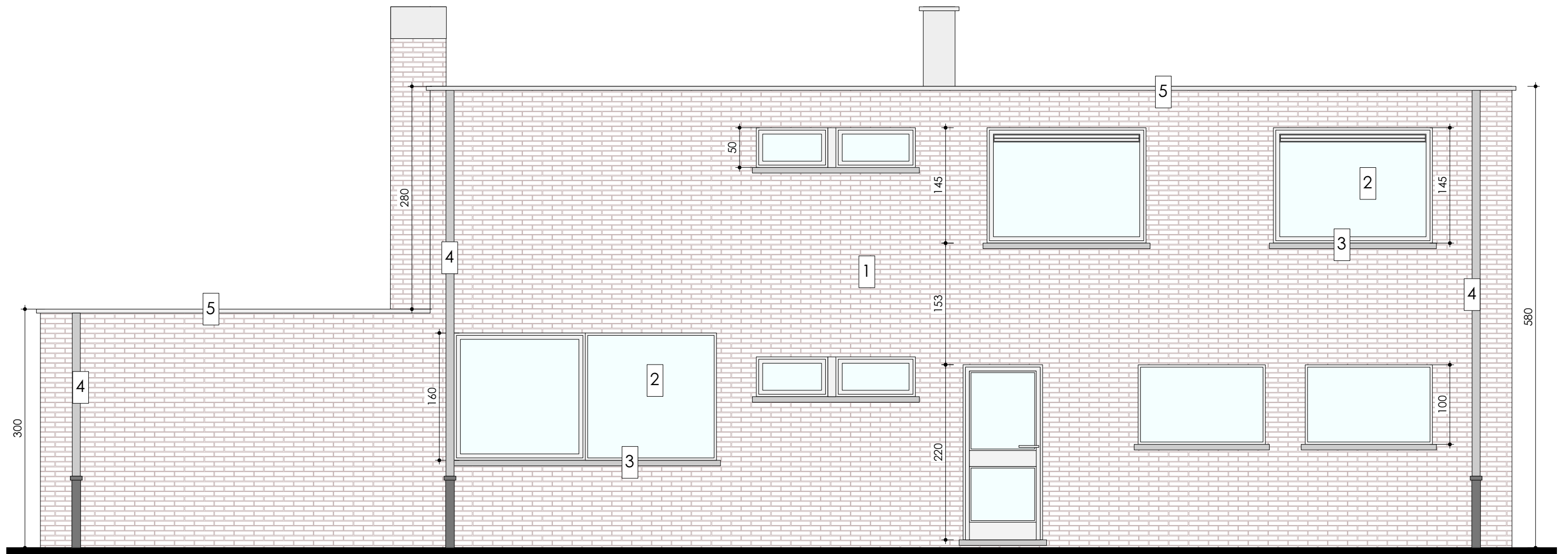
Linkerzijgevel-Bestaande toestand Schaal: 1:50
