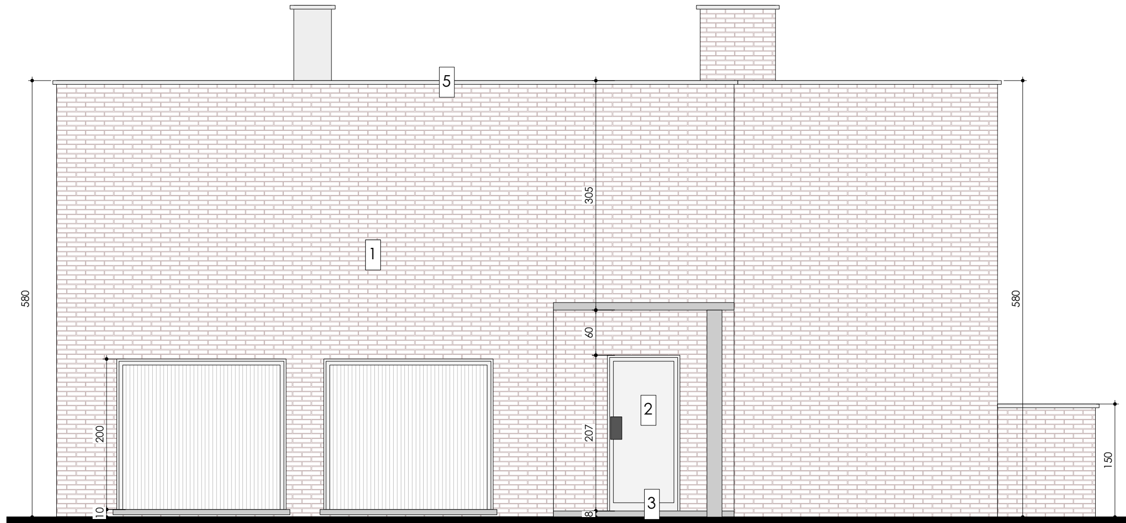
Voorgevel -Vergunde toestand Schaal: 1:50
